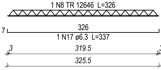
VT17a (8 unidades) (L17) ESC 1:50
