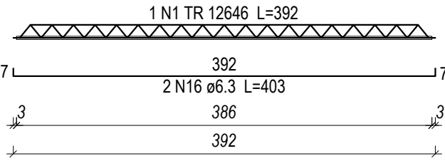
VT12a (13 unidades) (L12) ESC 1:50
