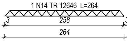
VT17a (8 unidades) (L17) ESC 1:50
