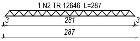
VT7a (14 unidades) (L7) ESC 1:50
