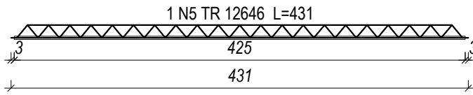
VT10a (5 unidades) (L10) ESC 1:50
