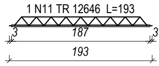
VT14a (11 unidades) (L14) ESC 1:50
