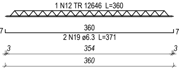
VT15a (11 unidades) (L15) ESC 1:50
