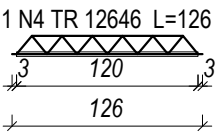
VT9a (6 unidades) (L9) ESC 1:50
