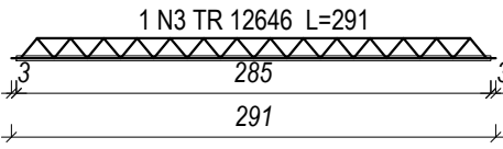
VT8a (14 unidades) (L8) ESC 1:50
