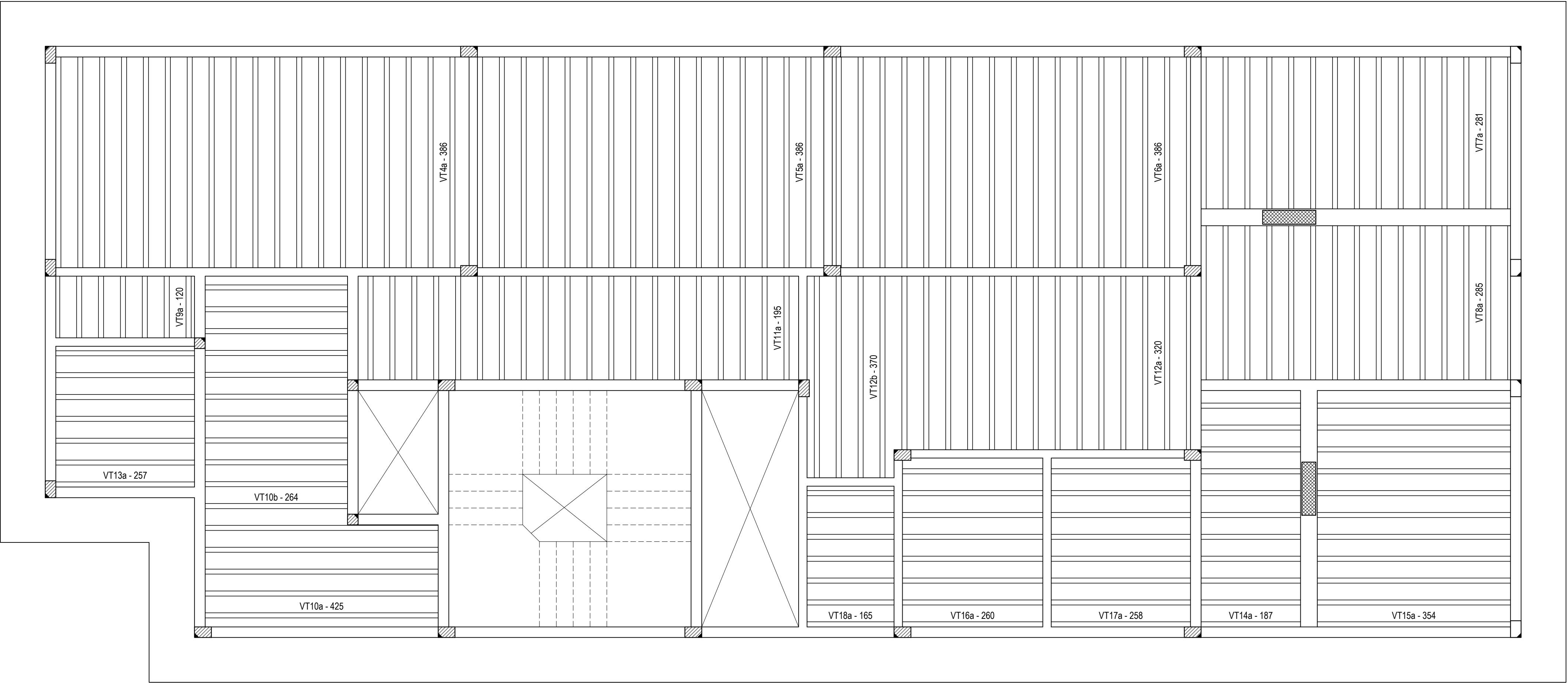
Planta de vigotas pré-moldadas do Segundo pavimento
