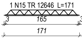
VT18a (7 unidades) (L18) ESC 1:50
