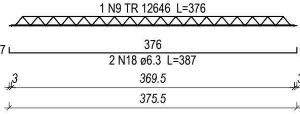
VT18a (7 unidades) (L18) ESC 1:50
