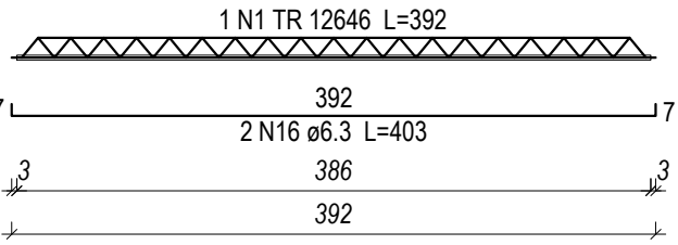
VT10b (11 unidades) (L10) ESC 1:50
