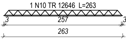
VT13a (7 unidades) (L13) ESC 1:50
