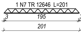
VT11a (20 unidades) (L11) ESC 1:50
