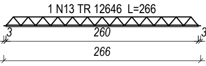
VT16a (8 unidades) (L16) ESC 1:50
