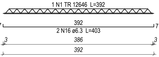
VT9a (6 unidades) (L9) ESC 1:50
