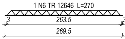
VT10b (11 unidades) (L10) ESC 1:50
